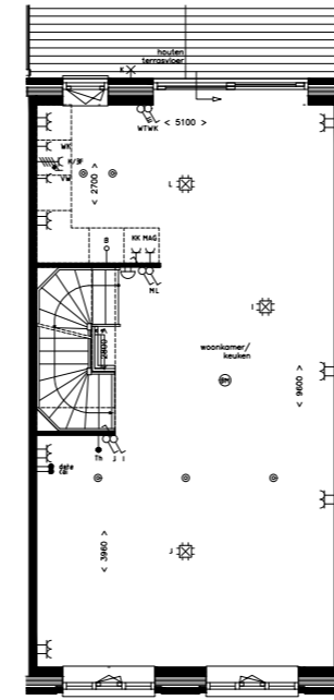
EERSTE VERDIEPING
