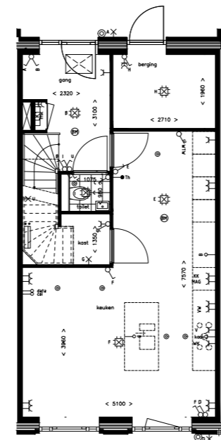
BEGANE GROND 00.038 KEUKEN VERPLAATSEN NAAR BEGANE GROND
