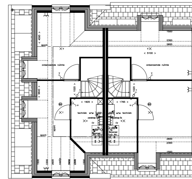
DERDE VERDIEPING 00.041 INDELING
