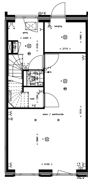
BEGANE GROND
