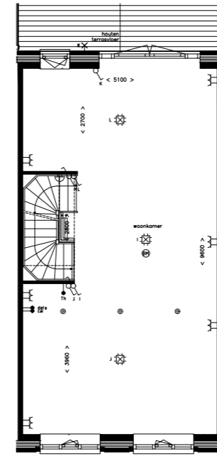
EERSTE VERDIEPING 00.038 KEUKEN VERPLAATSEN NAAR BEGANE GROND
