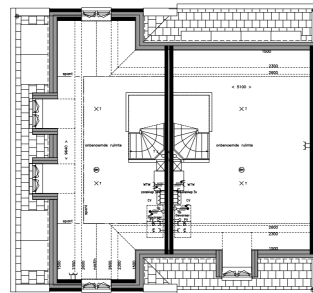
DERDE VERDIEPING
